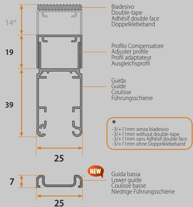
Sezione verticale - Vertical section Section verticale - Vertikaler Schnitt
