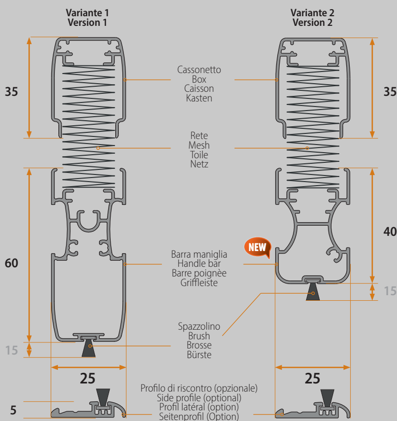
Sezione orizzontale - Horizontal section Section horizontale - Horizontaler Schnitt
